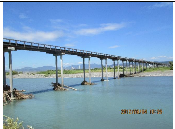
[2 日目巡検地 No,5]蓬莱橋…静岡県島田市にあり、大井川にかかる木造の橋。木造歩道橋としてはとても長くギネスブックに登録。幅は 2,4m、橋長はなんと 897m
